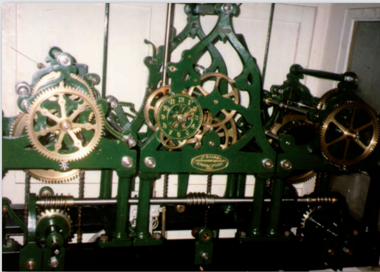
Uhrwerk im Turm der Pfarrkirche St. Blasius
